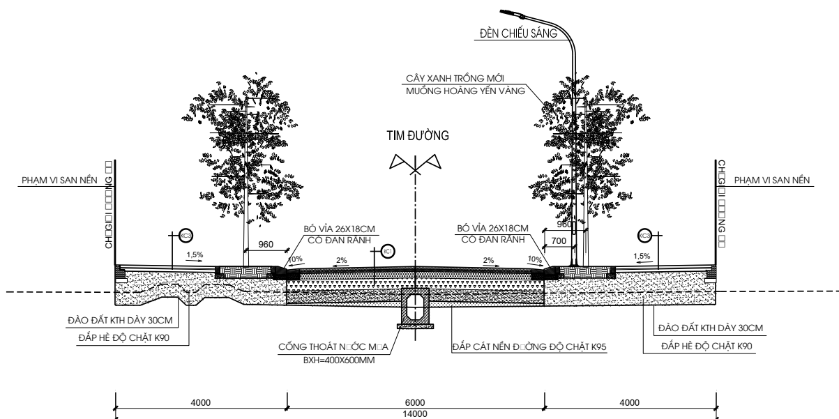
Hình 1. 5: Mặt cắt điển hình tuyến T3
