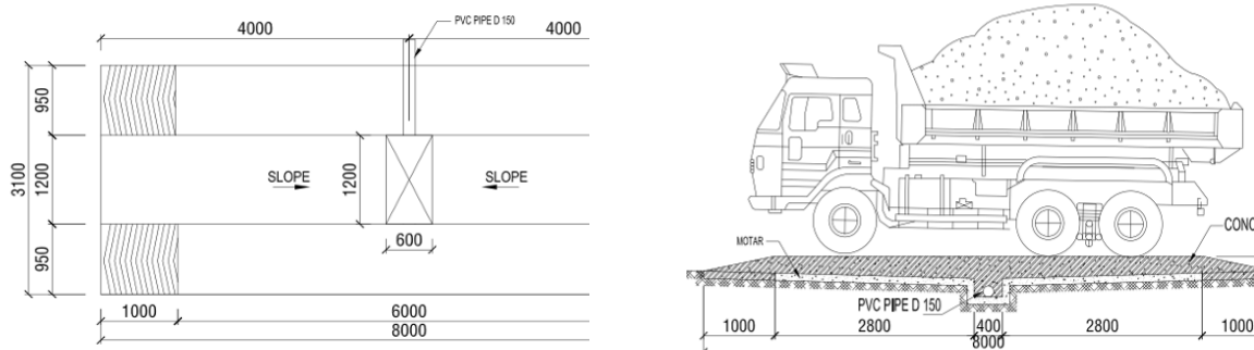
Hình 3. 2. Cấu tạo cầu rửa xe ra vào công trường
