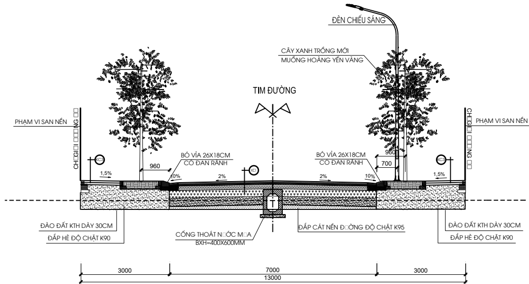
Hình 1. 4: Mặt cắt điển hình tuyến T2
