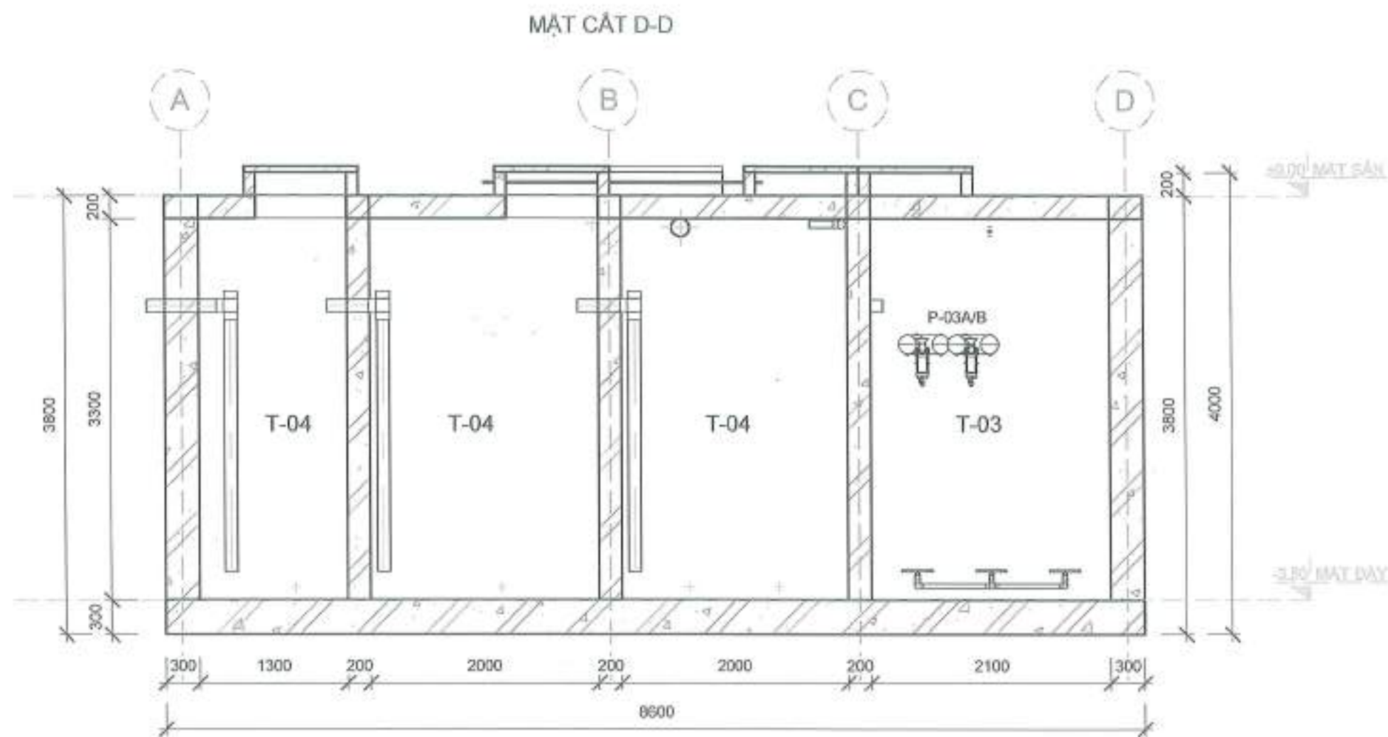
D-D MẶT CẮT D-D 1 : 40
