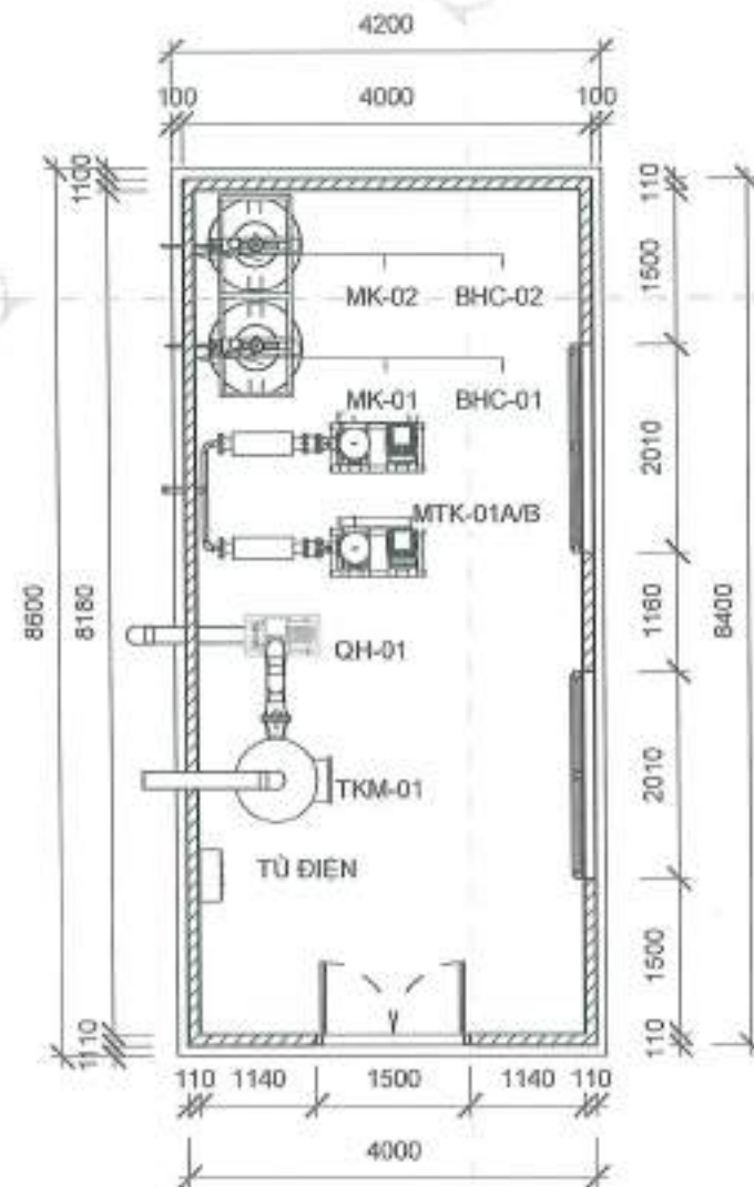
Mặt bằng nhà điều hành
