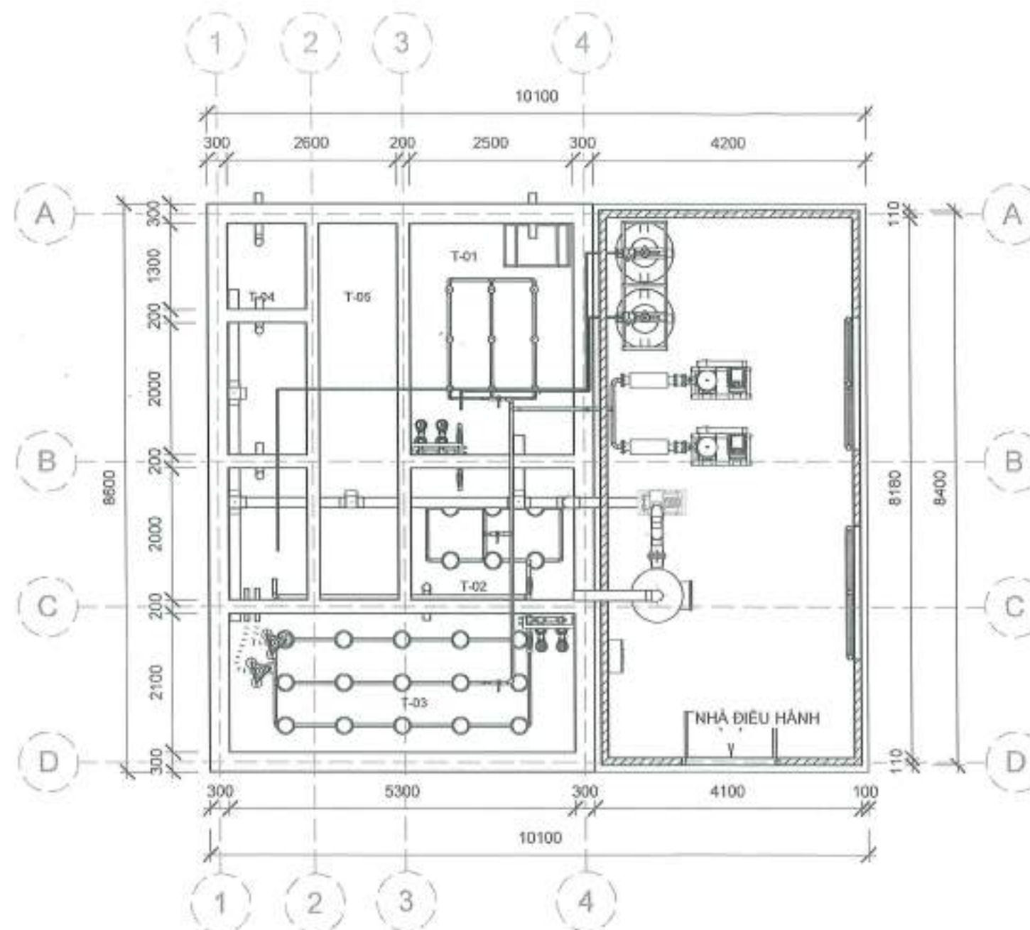
MẶT BẰNG BỐ TRÍ ĐƯỜNG ỐNG CÔNG NGHỆ TRẠM XLNT
