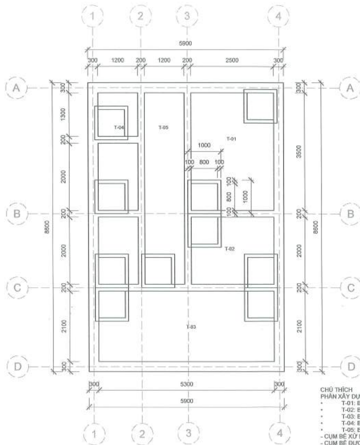
MẶT BẰNG BỐ TRÍ NẬP THẨM TRẠM XỬ LÝ NƯỚC THẢI
