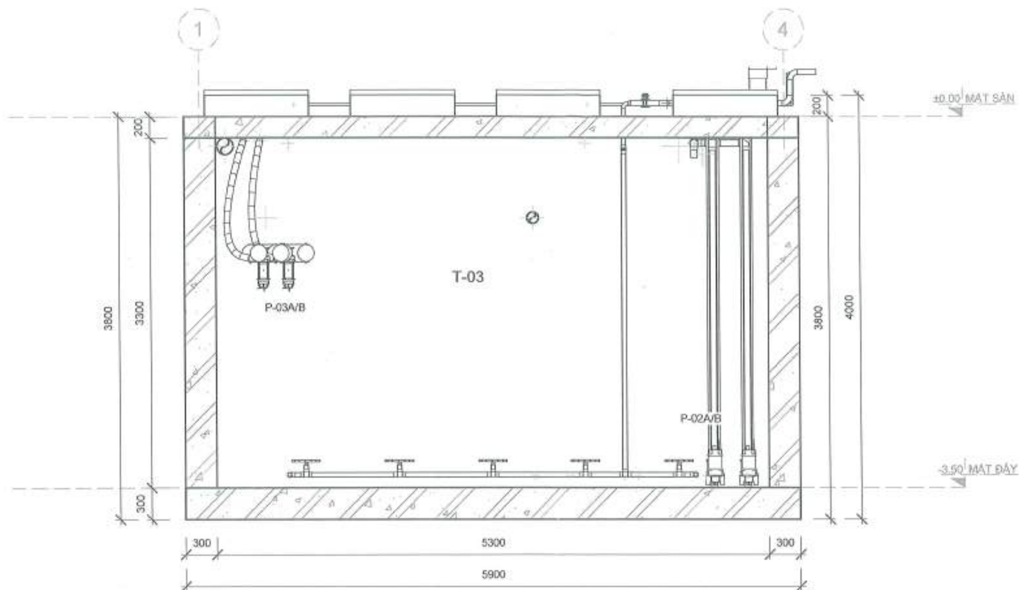
MẶT CẮT C-C 1 : 30
