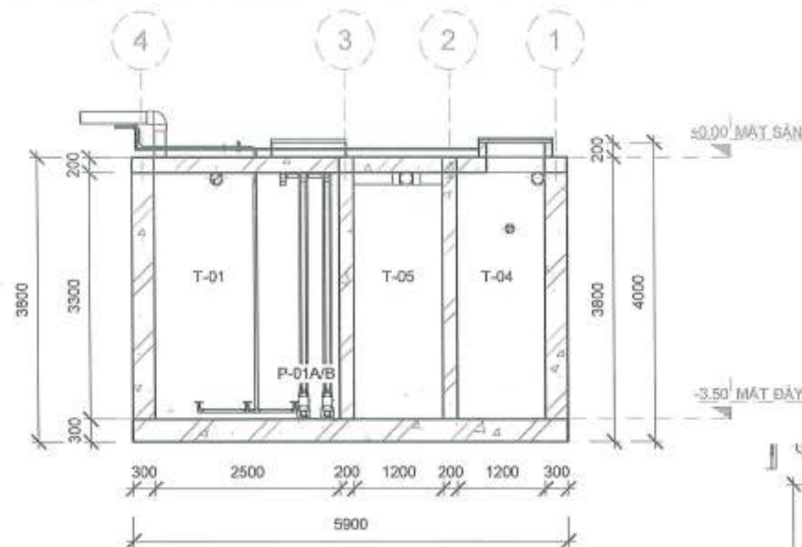
MẶT CẮT A-A 1 : 60
