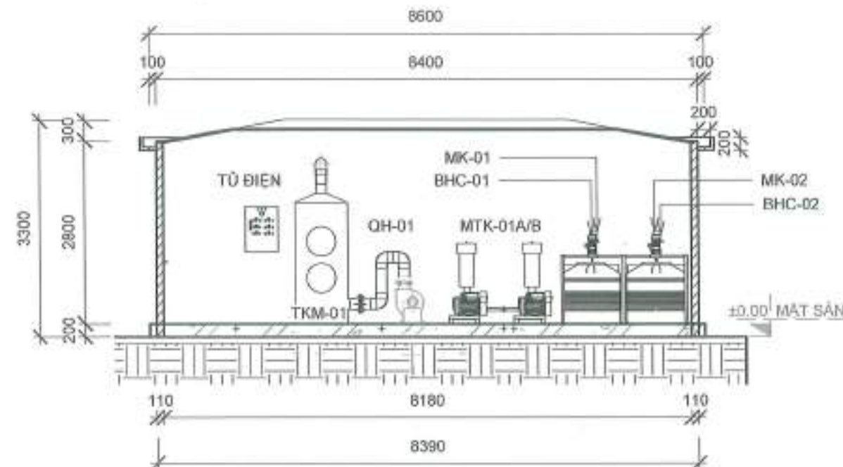
MẶT CẮT 1-1
