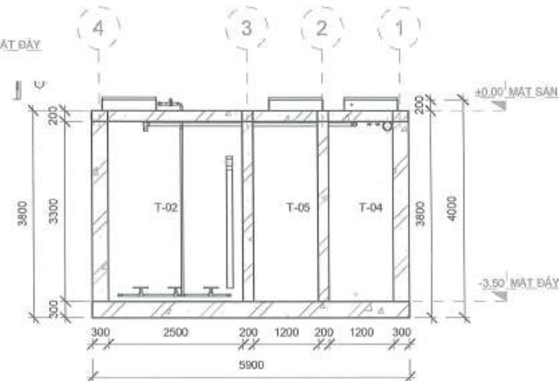
MẶT CẮT B-B 1 : 60
