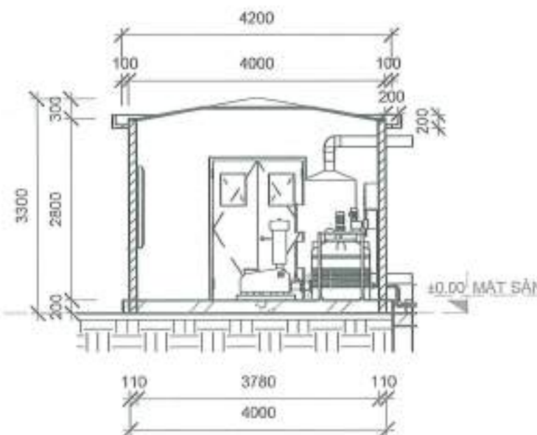
MẶT CẮT 2-2
