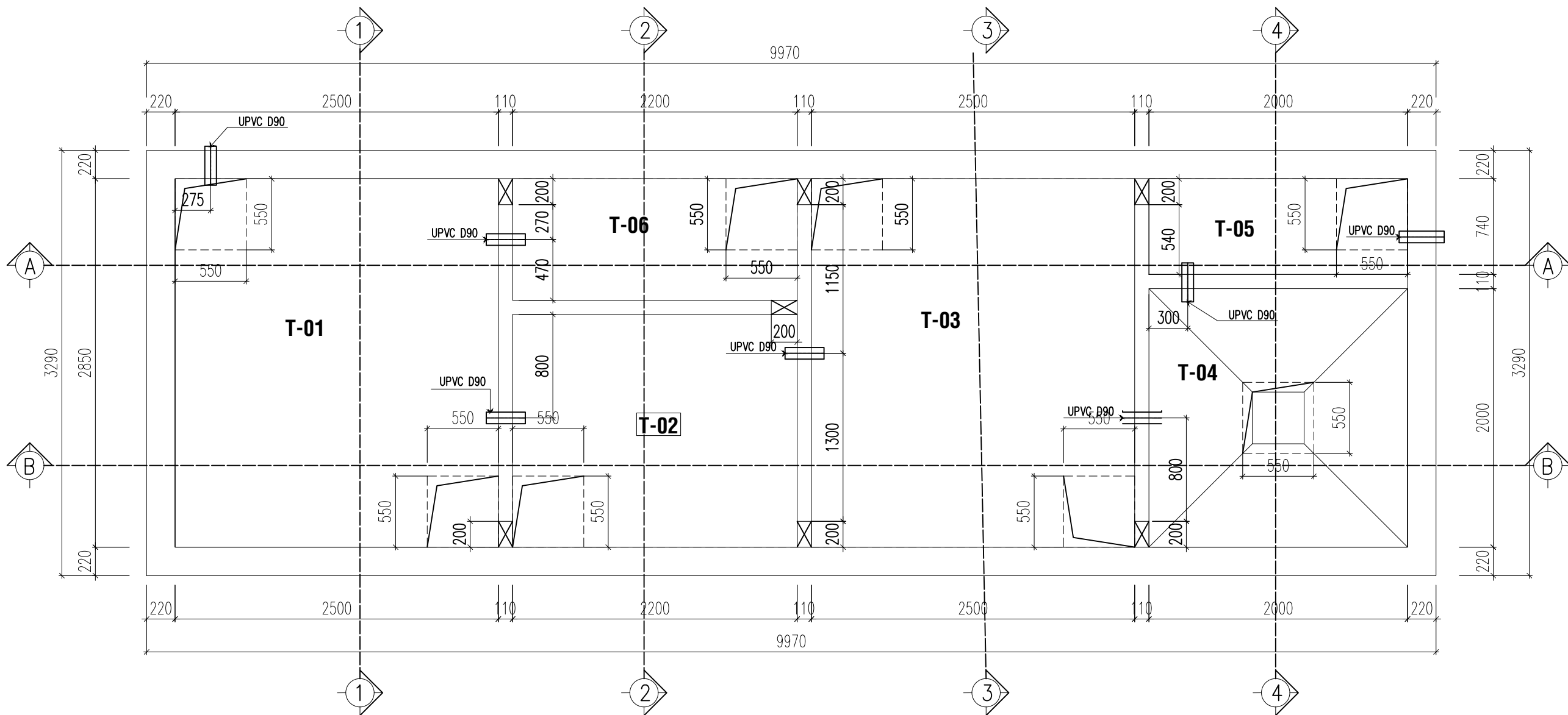
MẶT BẰNG LÔC CHỜ BỂ XỬ LÝ NƯỚC THẢI
