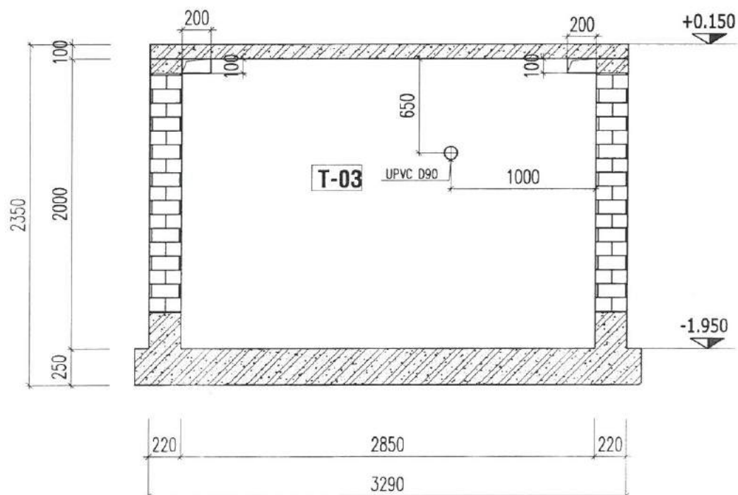
MẶT CẮT 3-3
