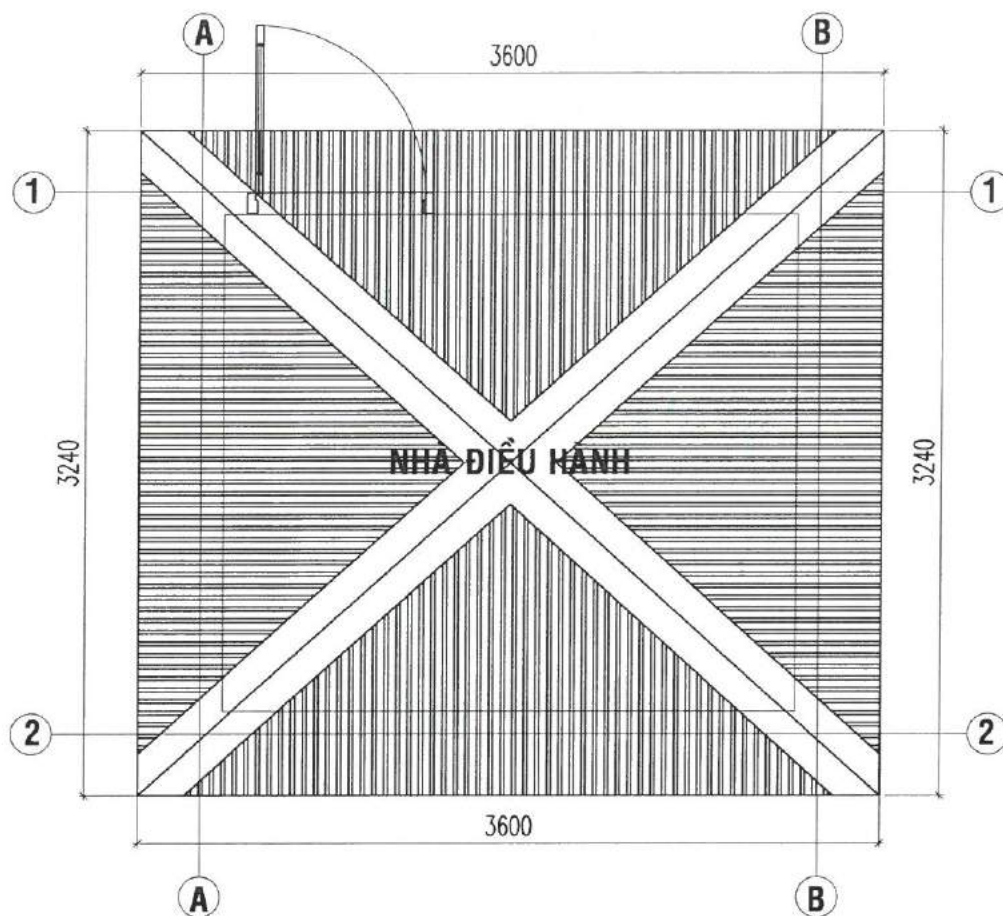
MẶT BẰNG MÁI NHÀ ĐIỀU HÀNH
