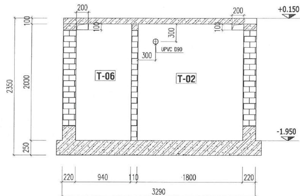
MẶT CẮT 2-2
