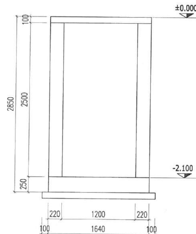
MẶT CẮT 1-1
