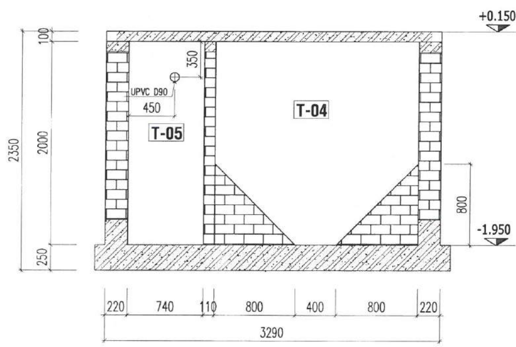
MẶT CẮT 4-4
