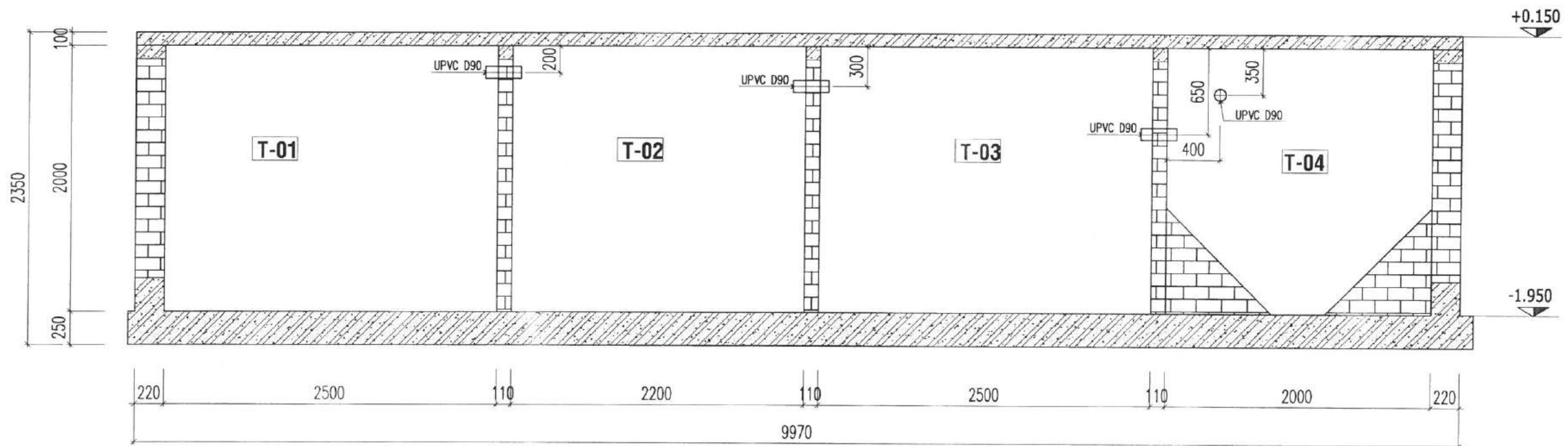
MẶT CẮT B-B
