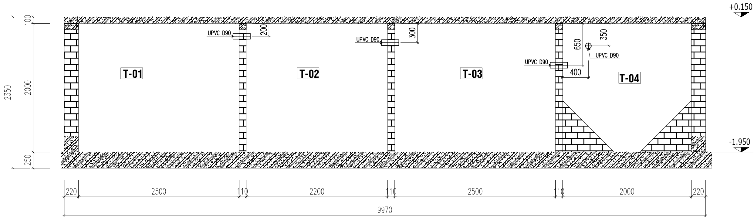
MẶT CẮT B-B
