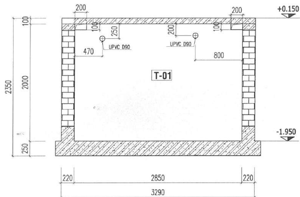
MẶT CẮT 1-1
