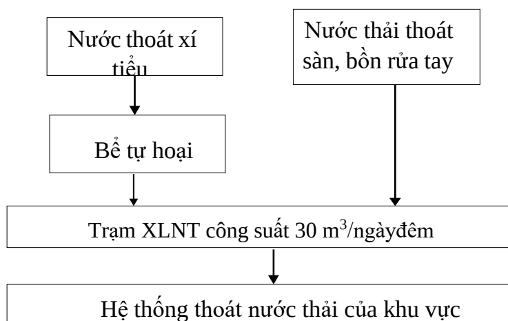
Hình 4. 2. Sơ đồ thu gom và xử lý nước thải sinh hoạt
