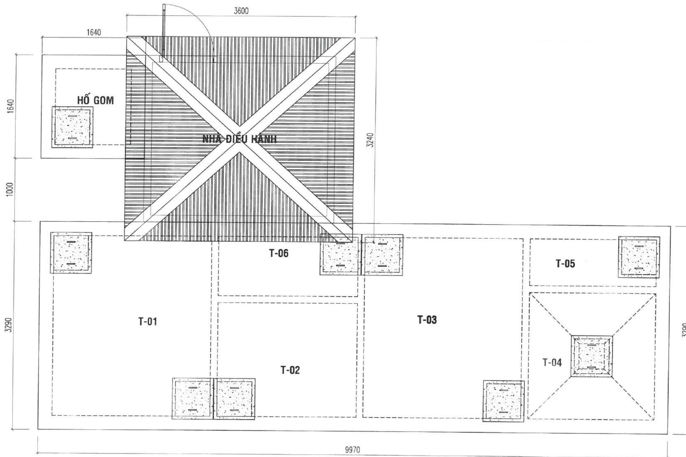
MẶT BẰNG TỔNG THỂ BỂ XỬ LÝ NƯỚC THẢI
