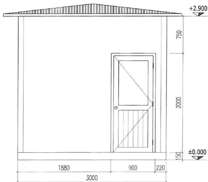
MẶT ĐỨNG TRỤC A-B
