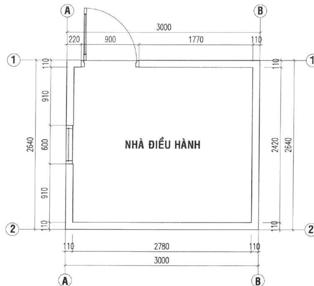
MẶT BẰNG NHÀ ĐIỀU HÀNH
