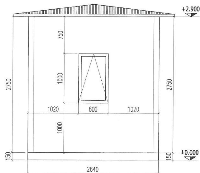
MẶT ĐỨNG TRỤC 1-2
