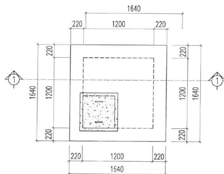
MẶT BẰNG
