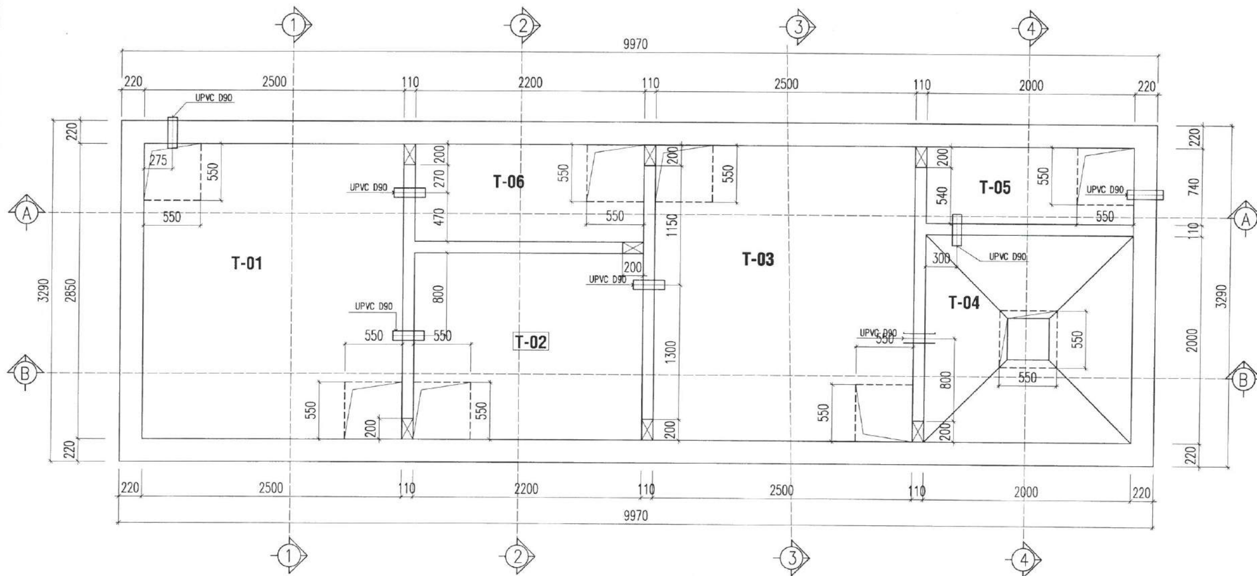
MẶT BẰNG LÔC CHỖ BỂ XỬ LÝ NƯỚC THẢI
