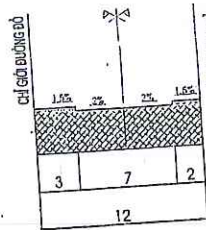
MẶT CẮT 1-1 Đất canh tác thôn Phúc Hậu 1
